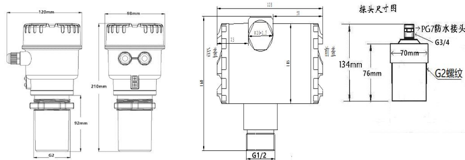
一体式规格尺寸 (图一)
