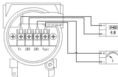
电压输出
