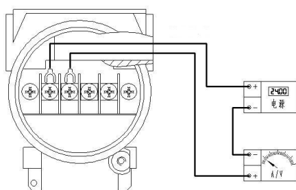
2 线电流输出
