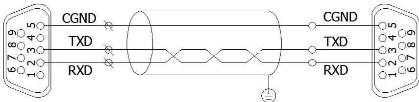
仪表侧RS232C通讯接口
