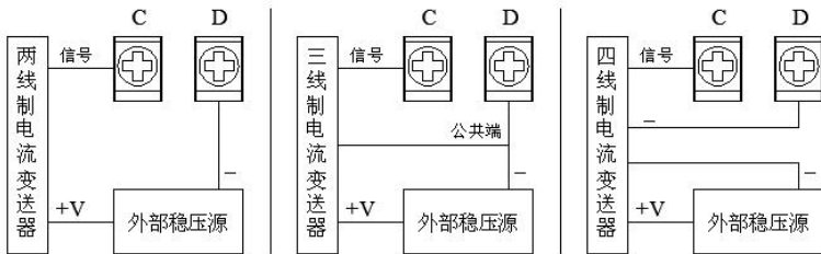
变送器接线方式(外接稳压源)
