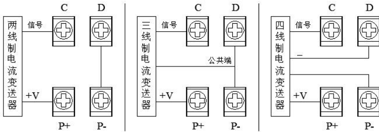
变送器接线方式(仪表馈电)
